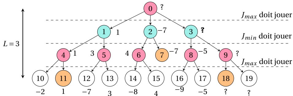
FIGURE 28.3 – L'élagage \alpha\beta permet sur cet exemple d'éviter l'exploration complète du sous-arbre du nœud numéro 3. En effet, comme c'est un nœud de J_{min} , que le premier nœud du niveau a un score de 1 et que le score calculé du nœud 8 vaut -5, alors on comprend que J_{min} remontera au moins -5 et que J_{max} ne choisira pas ce nœud numéro 3 car ce n'est pas le maximum du niveau.
