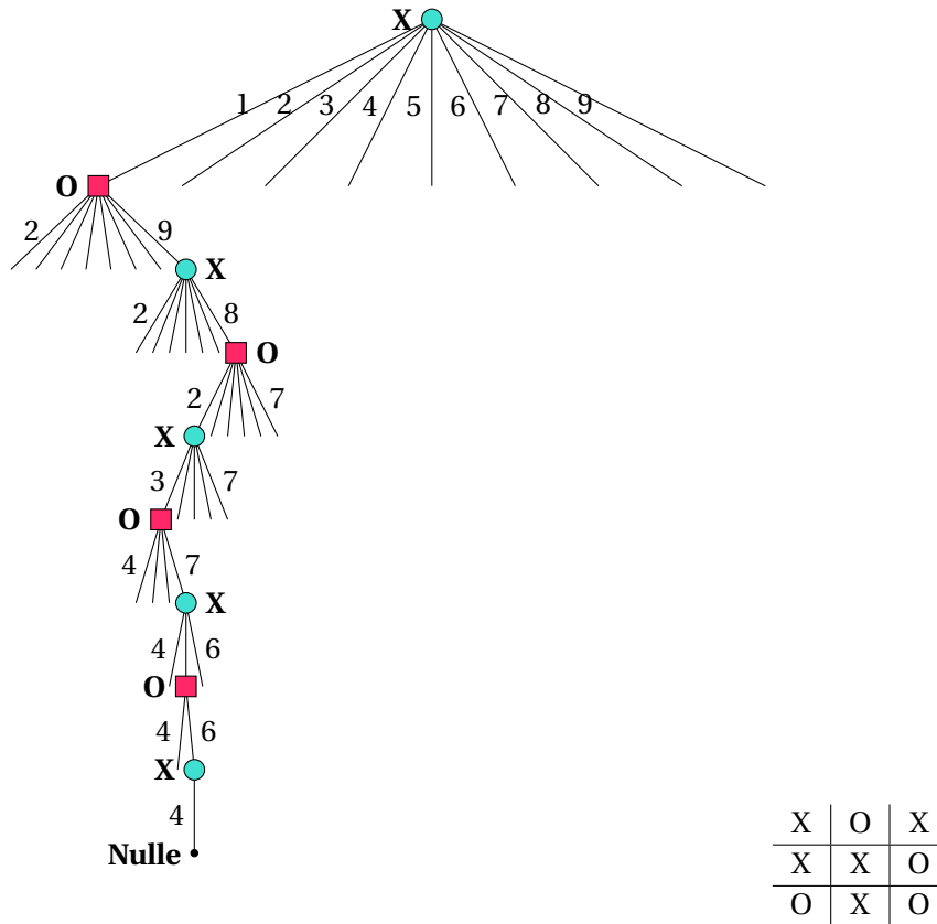
FIGURE 27.1 – Représentation partielle d’un arbre de jeu d’une partie de morpion. La feuille de l’arbre indique le résultat de la partie (nulle). Chaque nœud interne de l’arbre représente une position de X ou de O au cours de la partie dans laquelle les joueurs doivent faire un choix. On considère que les cases sont numérotées de 1 à 9 en ligne et en partant du haut. La position finale est donnée sous l’arbre. Le joueur à la croix X joue en premier car il contrôle la racine de l’arbre.
