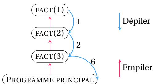
FIGURE 10.1 – Vision de la pile d’exécution de l’algorithme factoriel récursif 12 pour le calcul de 3!
