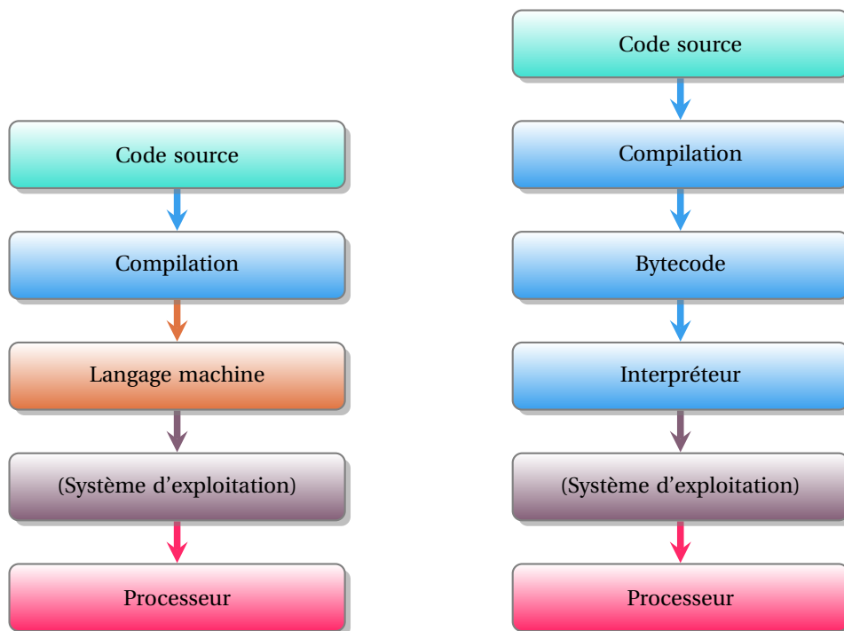
FIGURE 4.1 – Comparaison des chaînes d'exécution des langages compilés (à gauche) et des langages interprétés (à droite)
