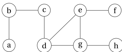
FIGURE 17.1 – Exemple de parcours en largeur au départ de a : a \rightarrow b \rightarrow c \rightarrow d \rightarrow e \rightarrow g \rightarrow f \rightarrow h .
