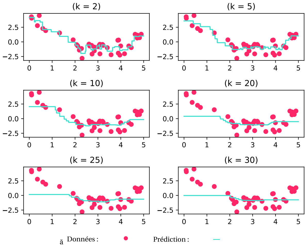
FIGURE 26.4 – Illustration de l'influence du nombre de voisins k sur une régression de modèle non linéaire dans le cadre de l'algorithme KNN
