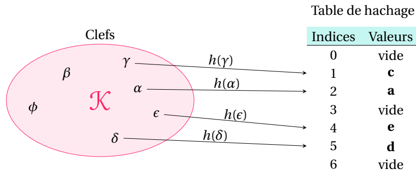
FIGURE 22.3 – Illustration de l’implémentation d’un dictionnaire par table de hachage. La fonction de hachage h permet de calculer les indices du tableau. La valeur a associée à \alpha se trouve à la case h(\alpha) du tableau. Toutes les clefs n’ont pas forcément de valeur associée à un moment donné de l’algorithme. Dans ce cas, à l’indice associé à cette clef, le tableau est vide.
