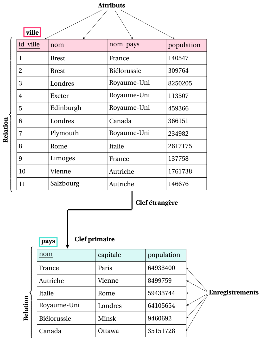
FIGURE 25.1 – Modèle relationnel utilisé pour les exemples de projection et de sélection.
