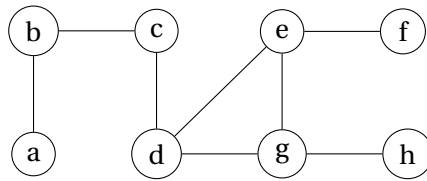
FIGURE 17.2 – Exemple de parcours en profondeur au départ de a : a \rightarrow b \rightarrow c \rightarrow d \rightarrow g \rightarrow h \rightarrow e \rightarrow f
