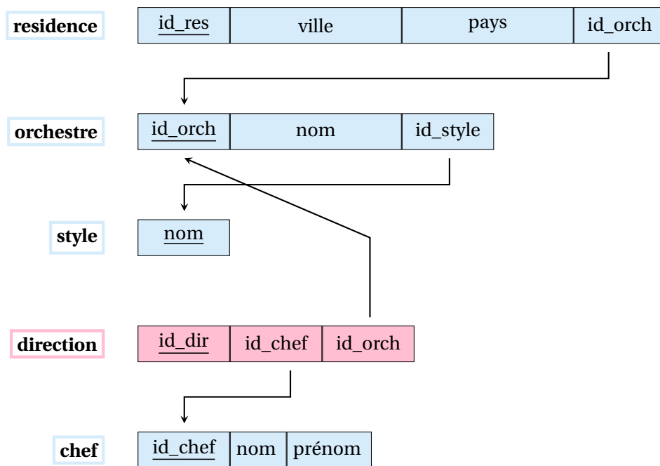
FIGURE 24.2 – Modèle relationnel construit à partir du modèle conceptuel 24.1. Seules les entêtes de colonne des relations sont représentées. Les associations du modèle conceptuel ont été intégrées aux tables en ajoutant des colonnes qui contiennent les clés primaires et les clés étrangères nécessaires ou en créant une nouvelle table ( direction ). Les flèches mettent en évidence ces associations.
