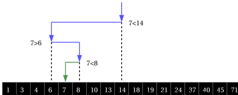
FIGURE 9.1 – Illustration de la recherche dichotomique de la valeur 7 dans un tableau trié (Source : Wikimedia Commons)
