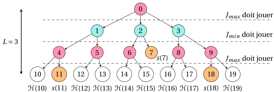
FIGURE 28.1 – Exemples d'arbre minimax. Chaque niveau est contrôlé par un seul joueur, J_{max} en rouge et J_{min} en cyan. La hauteur de l'arbre L est telle que seule une partie de l'arbre de jeu est accessible. Certaines feuilles sont visibles (en orange, c'est l'automne). L'arbre minimax s'achève donc parfois sur des nœuds internes pour lesquels on donne une estimation du gain (non coloré).
