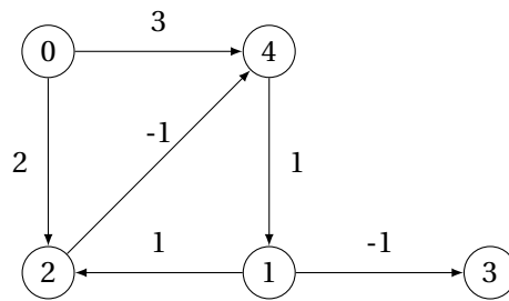
FIGURE 23.4 – Graphe orienté et pondéré pour application de l’algorithme de Bellman-Ford (sans cycle de pondération négative)
