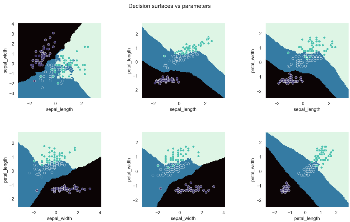
FIGURE 26.2 – Résultats de l'apprentissage de l'algorithme KNN sur le jeu de données de l'iris. Les régions de décisions du classificateur sont superposées aux valeurs vraies des espèces d'iris.
