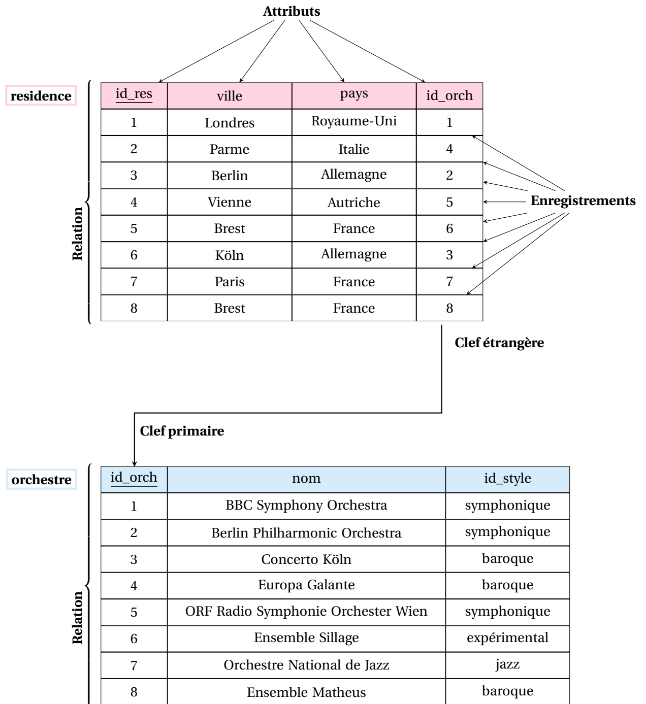
FIGURE 24.3 – Traduction d’une association de un à un dans un modèle relationnel. Modèle relationnel spécifiant les tables residence et orchestre du modèle relationnel de la figure 24.2.
