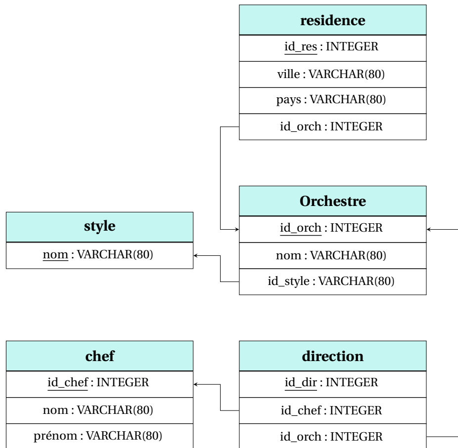
FIGURE 24.6 – Modèle physique de la base de données du modèle relationnel 24.2.
