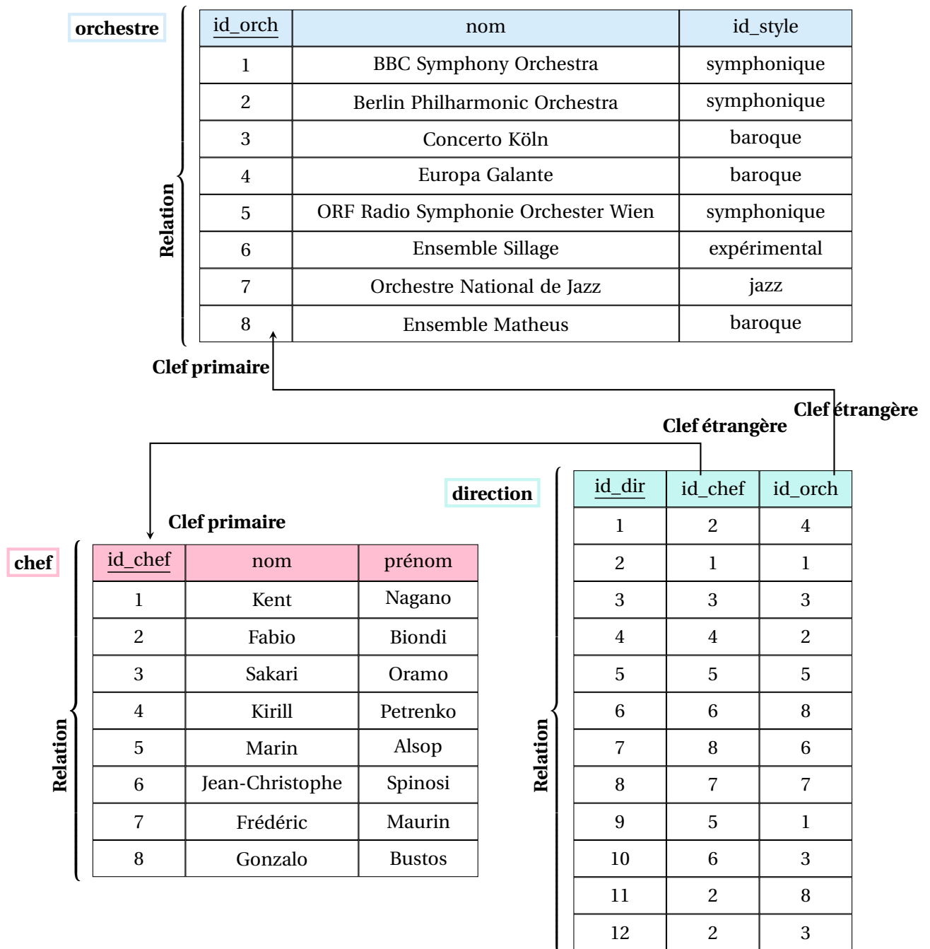
FIGURE 24.5 – Traduction d’une association de plusieurs à plusieurs dans un modèle relationnel. Modèle relationnel spécifiant les tables orchestre, direction et chef qui implémente l’association dirige du modèle conceptuel de la figure 24.1.
