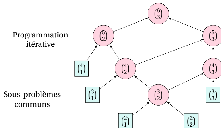
FIGURE 23.2 – Programmation itérative du calcul de \binom{6}{3} . Les rectangles correspondent à un cas terminal de la récursivité, les cercles à l’application de la formule récursive. Les sous-problèmes se chevauchent : par exemple, le calcul de \binom{3}{2} est utilisé par le calcul de \binom{4}{2} et \binom{4}{3} . En effectuant un calcul de bas en haut, l’idée est de ne le calculer qu’une seule fois ces éléments.
