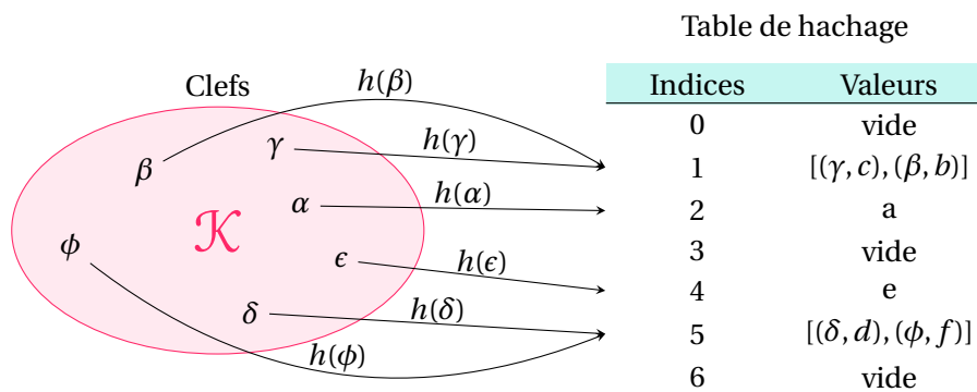
FIGURE 22.4 – Illustration de l’implémentation d’un dictionnaire par table de hachage avec chaînage. Les clefs \beta et \phi , engendrent des collisions. On stocke donc les valeurs possibles pour un même code (indice) dans une liste.
