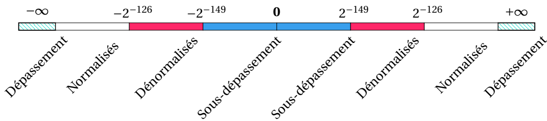
FIGURE 20.3 – Illustration de la répartition des nombres flottants IEEE754 en simple précision sur la droite des réels.
