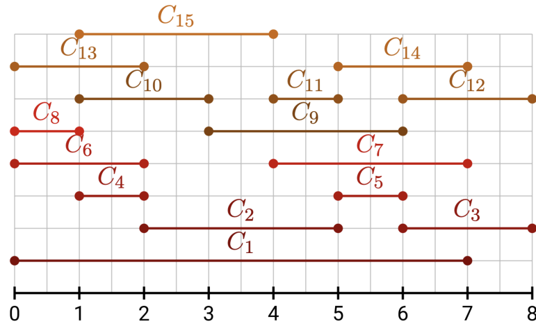
FIGURE 14.2 – Exemple de réservations de place au port correspondant à l'ensemble [[0, 7], [2, 5], [6, 8], [1, 2], [5, 6], [0, 2], [4, 7], [0, 1], [3, 6], [1, 3], [4, 5], [6, 8], [0, 2], [5, 7], [1, 4]]
