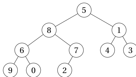
FIGURE 15.26 – Arbre binaire parfait
