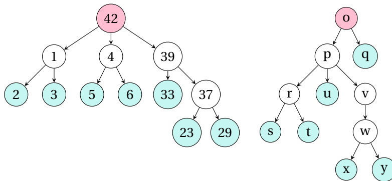
FIGURE 15.24 – Exemples d’arbres enracinés. Les racines des arbres sont en rouge, les feuilles en turquoise. Le tout forme une forêt.
