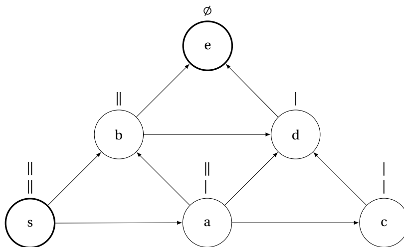
FIGURE 27.3 – Modélisation par graphe orienté d'une partie de jeu de Nim avec deux rangées de deux allumettes au départ. On peut jouer dessus avec un pion placé en s au départ. Puis chaque joueur fait avancer le pion d'un saut sur le graphe en sélectionnant un successeur en suivant les arcs. Le joueur qui se trouve en position e a gagné ou perdu dans la variante misère.
