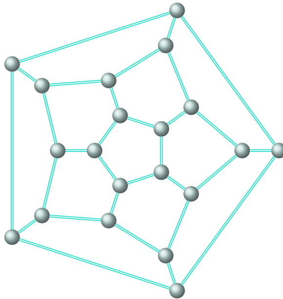
FIGURE 15.17 – Graphe du jeu icosien et du dodécahèdre (solide régulier à 12 faces pentagonales). C'est un graphe cubique car chaque sommet possède trois voisins. Ce graphe possède un cycle hamiltonien. Saurez-vous le trouver?
