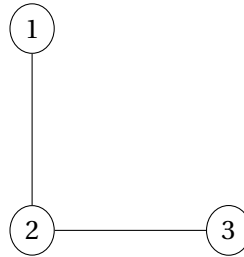
FIGURE 15.11 – Graphe d'ordre trois, de taille deux et de séquence [1, 1, 2]
