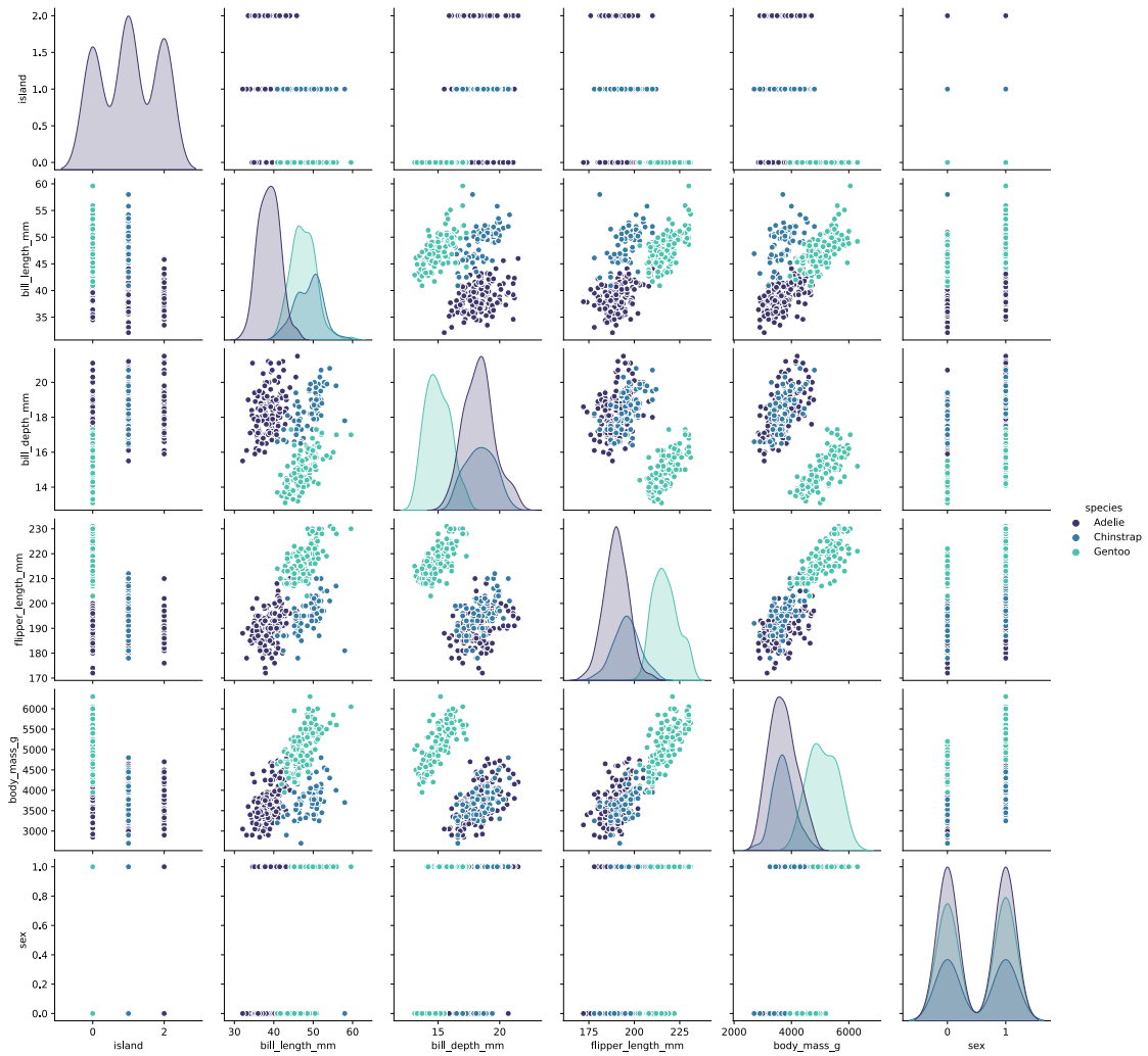
FIGURE 26.1 – Visualisation de la dispersion des paramètres sur le jeu de données des manchots répartis sur trois îles et en trois espèces
