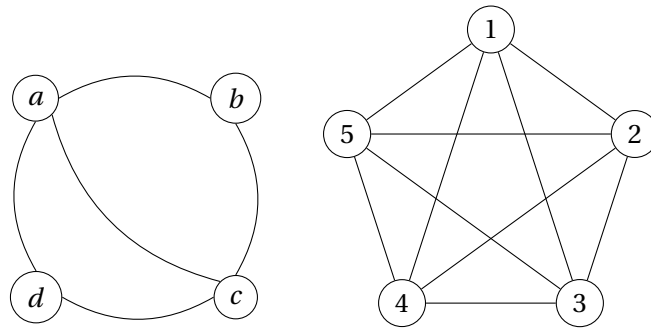
FIGURE 16.1 – Sur ces graphes, on peut vérifier les théorèmes de caractérisation des chaînes eulériennes et des cycles eulériens
