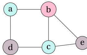
FIGURE 15.22 – Exemple de 3-coloration valide d'un graphe. Cette coloration est optimale.
