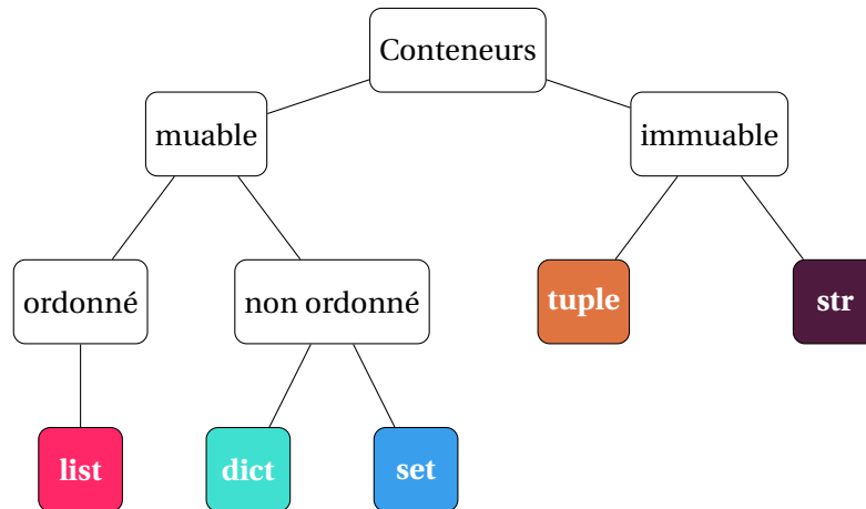
FIGURE 5.1 – Types de données composés du langage Python : les conteneurs
