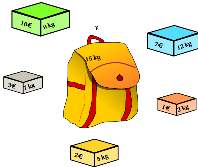
FIGURE 23.6 – Illustration du problème du sac à dos (d’après Wikipedia). On a cinq objets de poids 9, 12, 2, 7 et 5 kg et de valeur 10, 7, 1, 3 et 2 €. Le poids total admissible dans le sac est 15kg.
