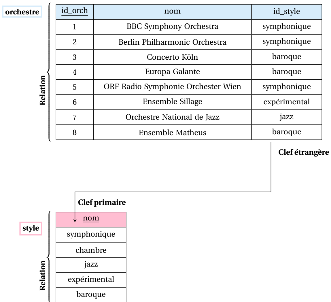
FIGURE 24.4 – Traduction d'une association de un à plusieurs dans un modèle relationnel. Modèle relationnel spécifiant les tables orchestre et style du modèle relationnel de la figure 24.2.
