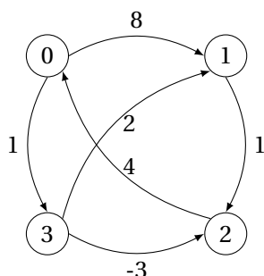
FIGURE 23.5 – Exemple de graphe orienté et pondéré pour expliquer le concept de matrice d'adjacence.
