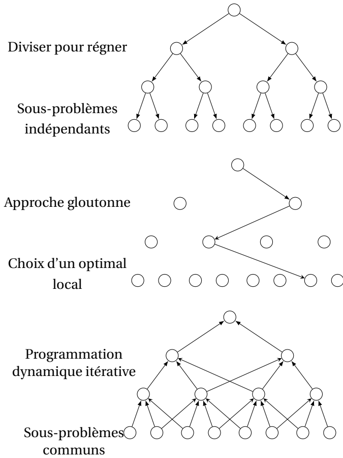
FIGURE 23.1 – Schématisation des différentes approches des algorithmes de décomposition d'un problème en sous-problèmes : diviser pour régner, approche gloutonne et programmation dynamique itérative.
