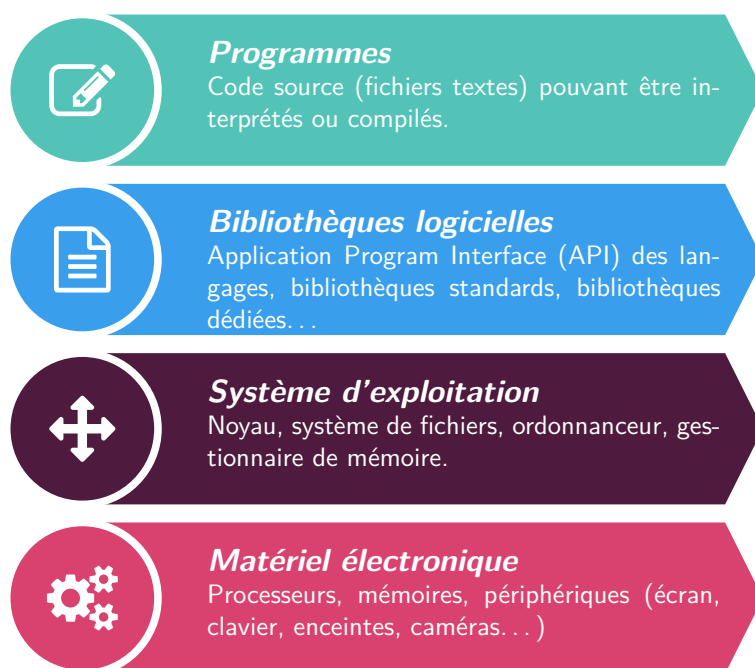
FIGURE 4.4 – Positionnement du système d'exploitation et des bibliothèques logicielles entre les éléments logiciels et le matériel électronique
