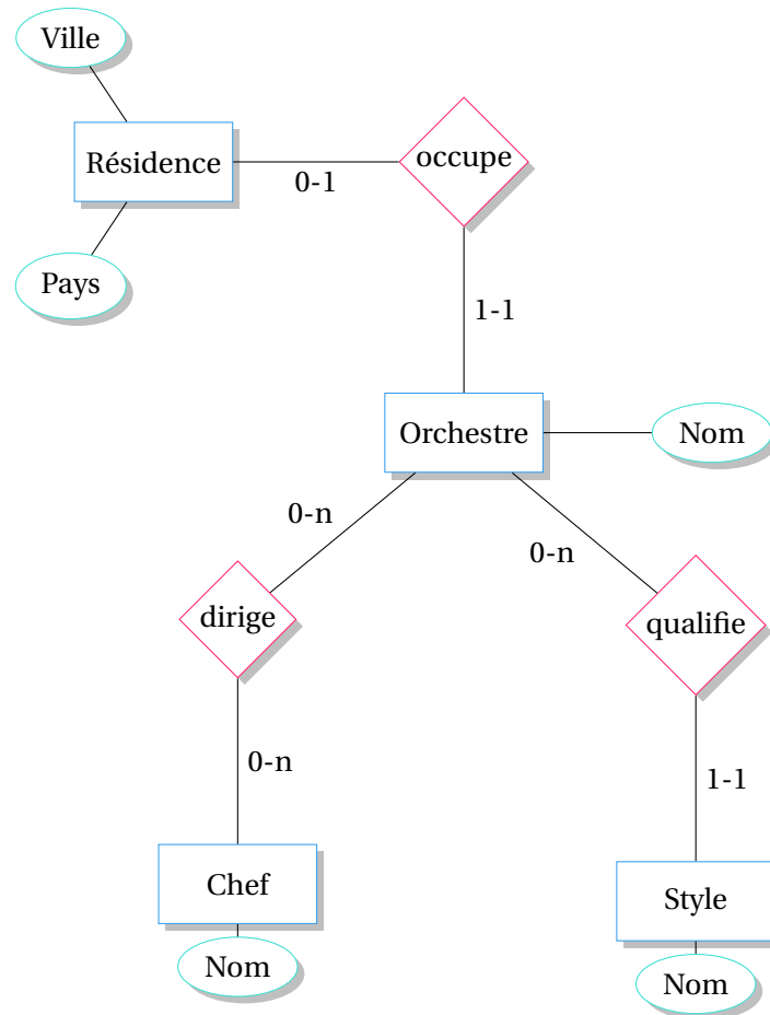
FIGURE 24.1 – Un modèle conceptuel de type entité-association associé à la réalité de l'exemple 103. Les entités sont inscrites dans des rectangles, les attributs des entités dans des ovales et les associations entre les entités dans des losanges. Des cardinalités sont précisées sur les arcs qui relient les entités aux associations
