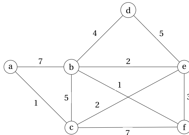
FIGURE 17.3 – Graphe pondéré à valeurs positives pour l’application de l’algorithme de Dijkstra.
