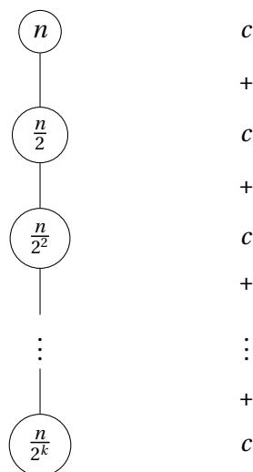
FIGURE 13.4 – Structure d'arbre et appels récursifs pour la récurrence de la recherche dichotomique : T(n) = T(n/2) + c . Hors appel récursif, la fonction opère un nombre constant d'opérations c indépendant de n en O(1) .
