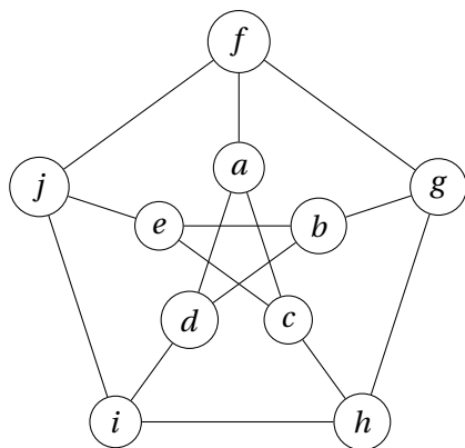
FIGURE 15.23 – Graphe de Petersen : saurez-vous proposer une coloration optimale de ce graphe sachant que son nombre chromatique vaut trois?
