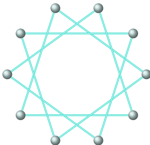
FIGURE 15.16 – Saurez-vous trouver le cycle eulérien de ce graphe?
