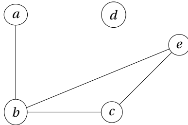
FIGURE 15.8 – Graphe d'ordre cinq, de taille quatre et de séquence [0, 1, 2, 2, 3] . Le sommet d est isolé. Ce graphe n'est ni complet ni connexe.
