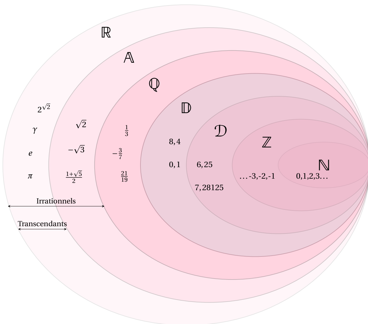
FIGURE 18.1 – Ensembles de nombres : naturels \mathbb{N} , relatifs \mathbb{Z} , dyadiques rationnels \mathcal{D} , décimaux \mathbb{D} , rationnels \mathbb{Q} , algébriques \mathbb{A} et réels \mathbb{R} .
