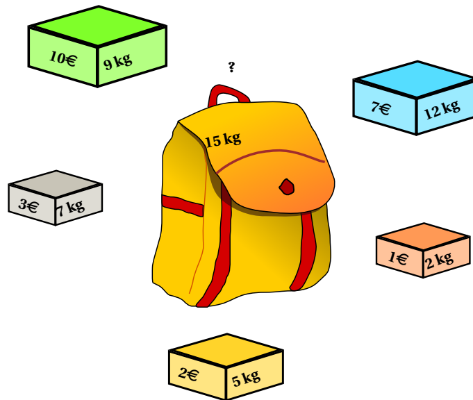
FIGURE 14.3 – Illustration du problème du sac à dos (d’après Wikipedia). On a cinq objets de poids 9, 12, 2, 7 et 5 kg et de valeur 10, 7, 1, 3 et 2. Le poids total admissible dans le sac est 15kg.
