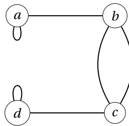
FIGURE 15.2 – Multigraphe à deux boucle et deux arêtes parallèles \dashrightarrow HORS PROGRAMME
