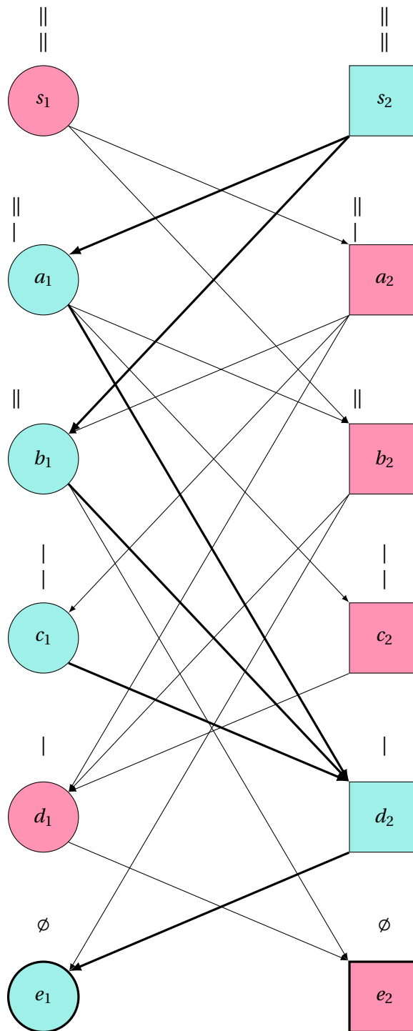
FIGURE 27.4 – Modélisation par graphe orienté biparti d'un jeu de Nim, variante misère : le dernier à jouer a perdu. Les sommets des joueurs 1 et 2 sont distingués par des cercles (1) et des carrés (2). La couleur cyan représente l'attracteur du joueur J_1 : \mathcal{A}_1 = \{s_2, a_1, b_1, c_1, d_2, e_1\} . On voit donc que 1 n'a pas intérêt à commencer à jouer dans cette configuration. Il en est de même pour le joueur 2 dont l'attracteur en rouge. C'est normal car la somme de Nim de la configuration initiale est nulle.
