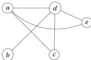
FIGURE 15.9 – Graphe complémentaire du graphe de la figure 15.8
