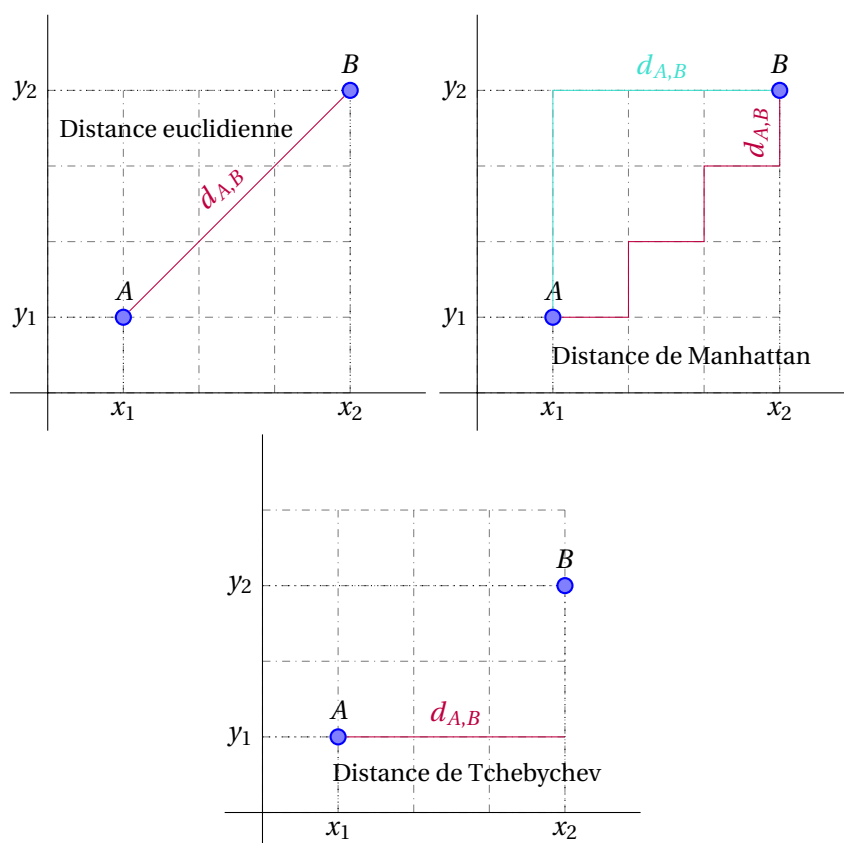
FIGURE 26.3 – Illustration des différentes distances dans le plan
