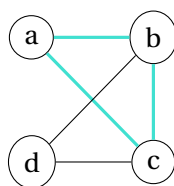
FIGURE 15.15 – Exemple de cycle en turquoise
