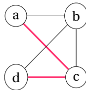
FIGURE 15.14 – Exemple de chaîne simple reliant a à d en rouge
