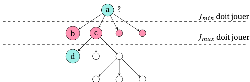
FIGURE 28.5 – L'élagage \beta : supposons que S(b) ait déjà été calculé par l'algorithme Minimax. Si S(b) \leq S(d) , alors il est inutile d'explorer le sous-arbre c : J_{min} ne choisira pas le nœud c , il lui préférera b .
