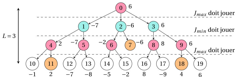
FIGURE 28.2 – Exemples d'arbre minimax complété avec les scores. Chaque niveau est contrôlé par un seul joueur, J_{max} en rouge et J_{min} en cyan.
