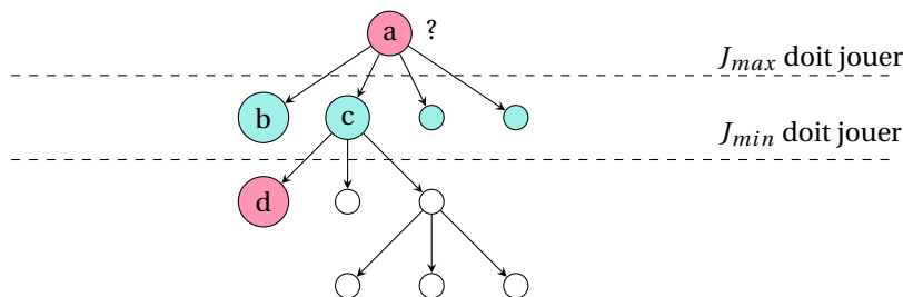
FIGURE 28.4 – L'élagage \alpha : supposons que S(b) ait déjà été calculé par l'algorithme Minimax. Si S(b) \geq S(d) , alors il est inutile d'explorer le sous-arbre c : J_{max} ne choisira pas le nœud c , il lui préférera b .
