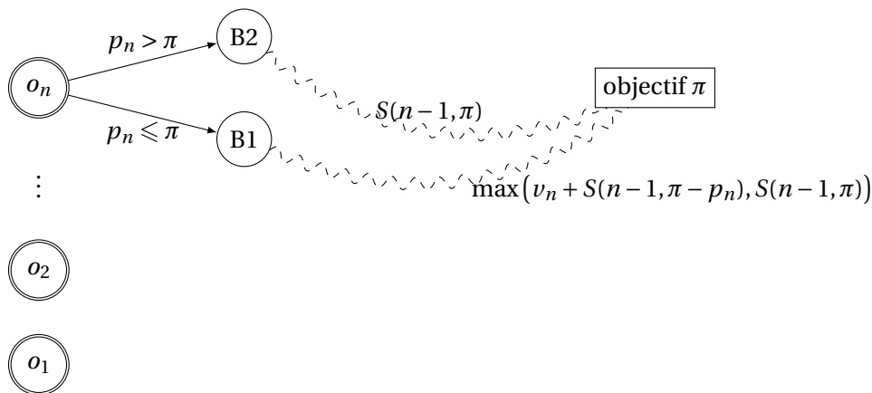
FIGURE 23.7 – Formulation récursive du problème du sac à dos.
