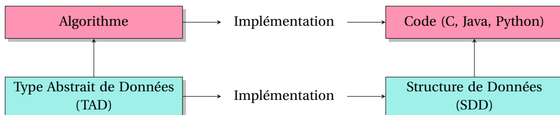
FIGURE 1.1 – Imbrication des concepts d'algorithme, de type abstrait de données, d'implémentation, de code et de structure de données
