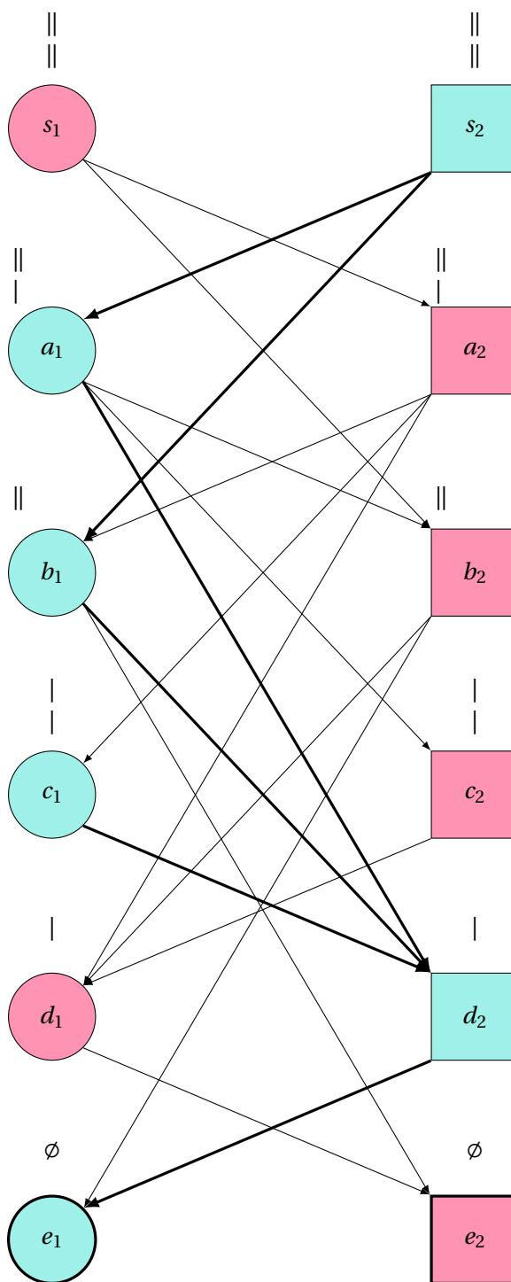
FIGURE 26.4 – Modélisation par graphe orienté biparti d'un jeu de Nim, variante misère : le dernier à jouer a perdu. Les sommets des joueurs 1 et 2 sont distingués par des cercles (1) et des carrés (2). La couleur cyan représente l'attracteur du joueur J_1 : \mathcal{A}_1 = \{s_2, a_1, b_1, c_1, d_2, e_1\} . On voit donc que 1 n'a pas intérêt à commencer à jouer dans cette configuration. Il en est de même pour le joueur 2 dont l'attracteur en rouge. C'est normal car la somme de Nim de la configuration initiale est nulle.
