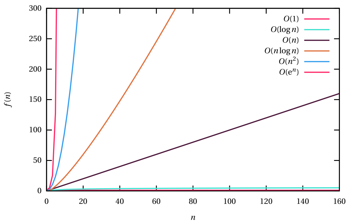
FIGURE 12.1 – Comparaison des croissances des complexités usuelles
