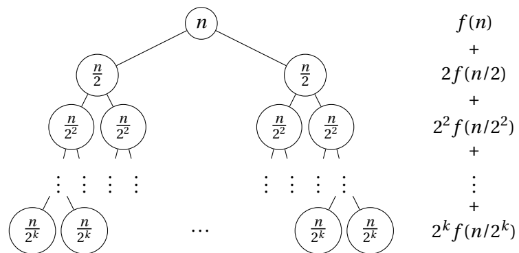
FIGURE 12.5 – Structure d'arbre et appels récursifs pour le tri fusion : T(n) = 2T(n/2) + f(n) et \frac{n}{2^k} = 1 . La fonction FUSION opère un nombre d'opérations f(n) .
