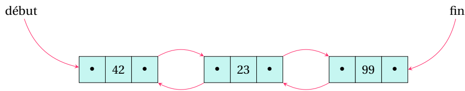
FIGURE 10.3 – Représentation d’une liste doublement chaînée d’entiers L . On conserve un pointeur sur le premier élément et un autre sur le dernier élément de la liste.
