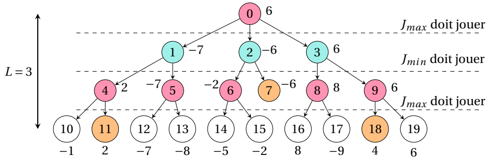
FIGURE 26.6 – Exemples d’arbre minimax complété avec les scores. Chaque niveau est contrôlé par un seul joueur, J_{max} en rouge et J_{min} en cyan.
