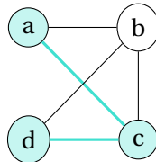
FIGURE 14.20 – Exemple de sous-graphe induit par les sommets S = \{a, c, d\} en turquoise. G[S] = (S = \{a, c, d\}, A = \{ac, cd\})
