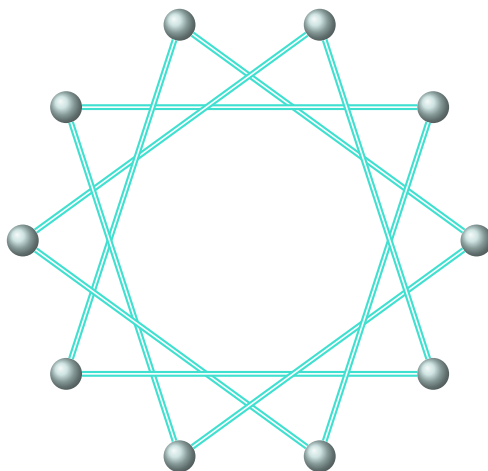
FIGURE 14.16 – Saurez-vous trouver le cycle eulérien de ce graphe?
