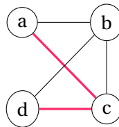
FIGURE 14.14 – Exemple de chaîne simple reliant a à d en rouge
