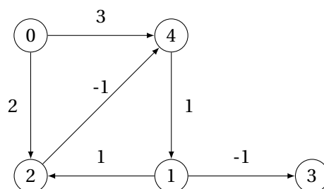
FIGURE 22.4 – Graphe orienté et pondéré pour application de l'algorithme de Bellman-Ford (sans cycle de pondération négative)
