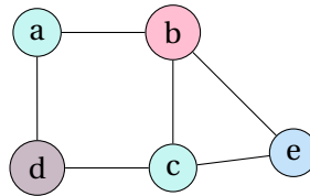
FIGURE 14.21 – Exemple de 4-coloration valide d'un graphe. Cette coloration n'est pas optimale.
