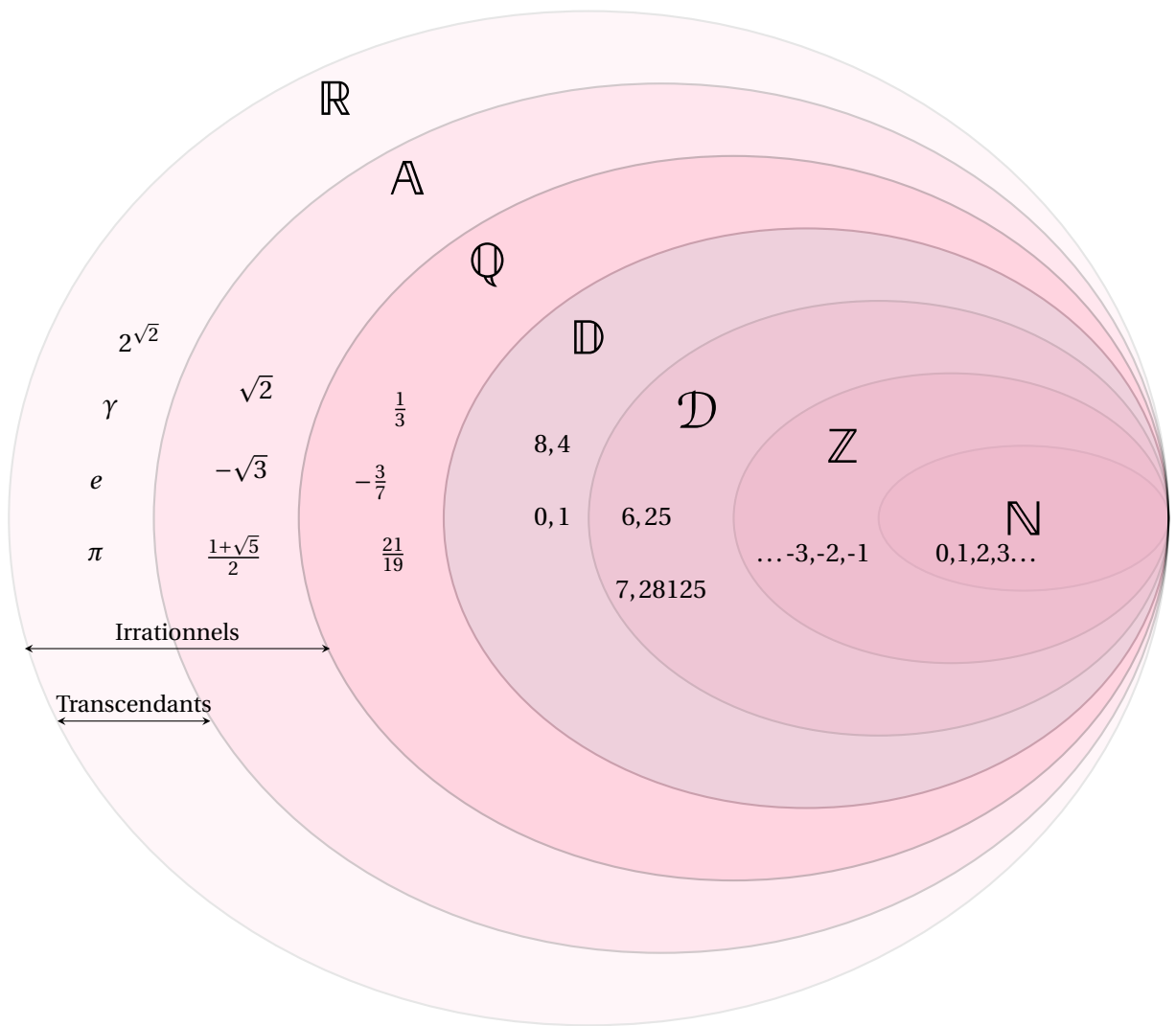
FIGURE 17.1 – Ensembles de nombres : naturels \mathbb{N} , relatifs \mathbb{Z} , dyadiques rationnels \mathcal{D} , décimaux \mathbb{D} , rationnels \mathbb{Q} , algébriques \mathbb{A} et réels \mathbb{R} .
