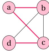
FIGURE 14.19 – Exemple de sous-graphe couvrant G en rouge : G = (S = \{a, b, c, d\}, A = \{ab, ac, cd\})
