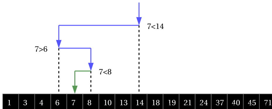
FIGURE 8.1 – Illustration de la recherche dichotomique de la valeur 7 dans un tableau trié (Source : Wikimedia Commons)
