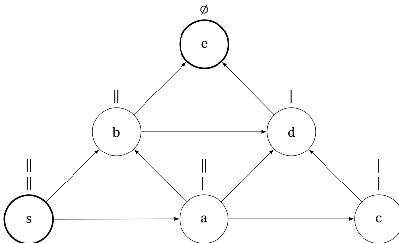
FIGURE 26.3 – Modélisation par graphe orienté d'une partie de jeu de Nim avec deux rangées de deux allumettes au départ. On peut jouer dessus avec un pion placé en s au départ. Puis chaque joueur fait avancer le pion d'un saut sur le graphe en sélectionnant un successeur en suivant les arcs. Le joueur qui se trouve en position e a gagné ou perdu dans la variante misère.
