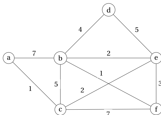
FIGURE 16.3 – Graphe pondéré à valeurs positives pour l’application de l’algorithme de Dijkstra.
