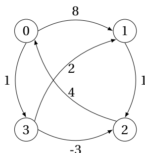
FIGURE 22.5 – Exemple de graphe orienté et pondéré pour expliquer le concept de matrice d'adjacence.
