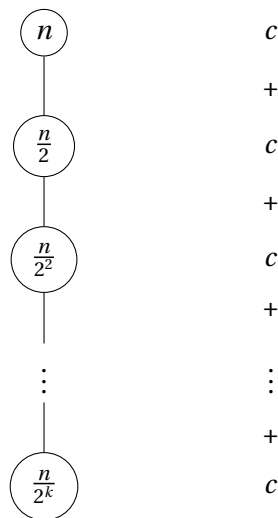
FIGURE 12.4 – Structure d'arbre et appels récursifs pour la récurrence de la recherche dichotomique : T(n) = T(n/2) + c . Hors appel récursif, la fonction opère un nombre constant d'opérations c indépendant de n en O(1) .
