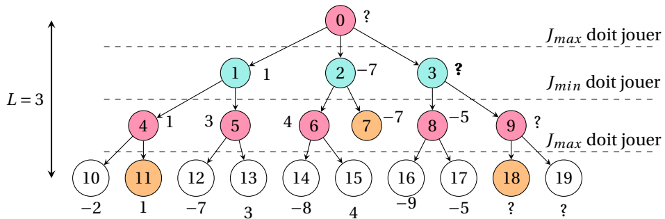
FIGURE 26.7 – L’élagage \alpha\beta permet sur cet exemple d’éviter l’exploration complète du sous-arbre du nœud numéro 3. En effet, comme c’est un nœud de J_{min} , que le premier nœud du niveau a un score de 1 et que le score calculé du nœud 8 vaut -5, alors on comprend que J_{min} remontera au moins -5 et que J_{max} ne choisira pas ce nœud numéro 3 car ce n’est pas le maximum du niveau.
