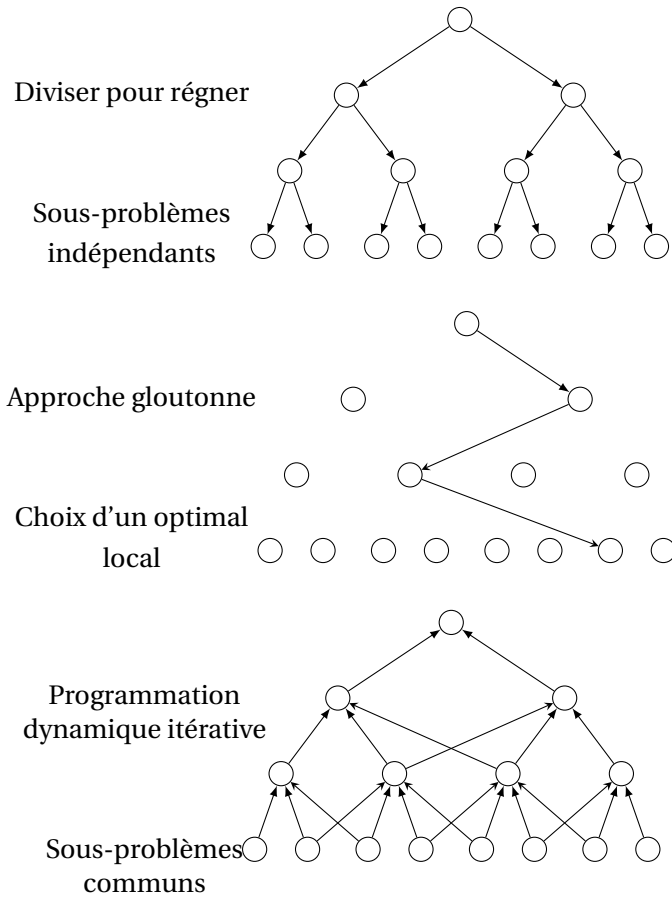
FIGURE 22.1 – Schématisation des différentes approches des algorithmes de décomposition d'un problème en sous-problèmes : diviser pour régner, approche gloutonne et programmation dynamique itérative.
