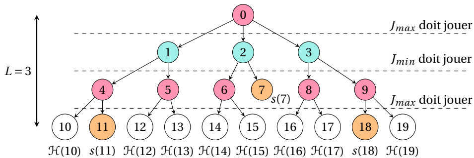
FIGURE 26.5 – Exemples d'arbre minimax. Chaque niveau est contrôlé par un seul joueur, J_{max} en rouge et J_{min} en cyan. La hauteur de l'arbre L est telle que seule une partie de l'arbre de jeu est accessible. Certaines feuilles sont visibles (en orange, c'est l'automne). L'arbre minimax s'achève donc parfois sur des nœuds internes pour lesquels on donne une estimation du gain (non coloré).
