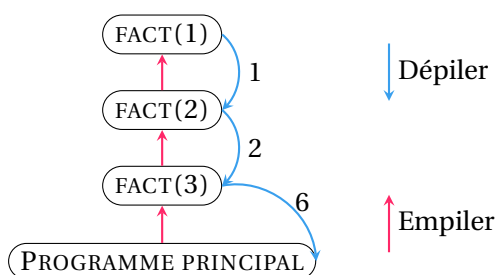
FIGURE 9.1 – Vision de la pile d’exécution de l’algorithme factoriel récursif 12 pour le calcul de 3!
