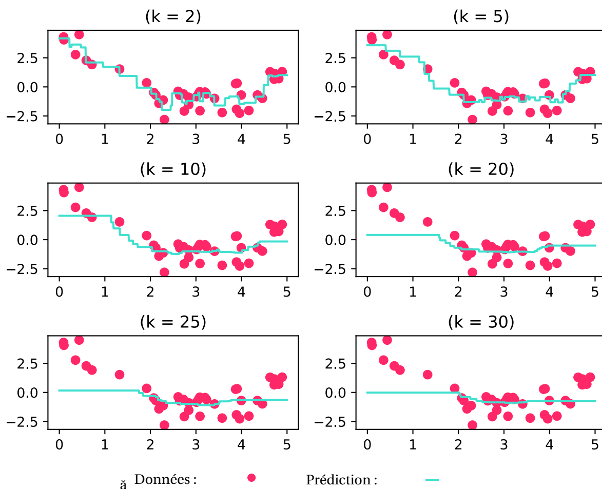
FIGURE 25.4 – Illustration de l'influence du nombre de voisins k sur une régression de modèle non linéaire dans le cadre de l'algorithme KNN
