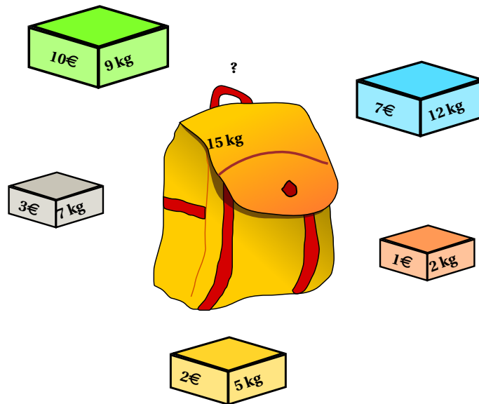
FIGURE 13.3 – Illustration du problème du sac à dos (d’après Wikipedia). On a cinq objets de poids 9, 12, 2, 7 et 5 kg et de valeur 10, 7, 1, 3 et 2. Le poids total admissible dans le sac est 15kg.
