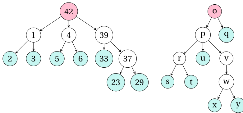
FIGURE 14.24 – Exemples d’arbres enracinés. Les racines des arbres sont en rouge, les feuilles en turquoise. Le tout forme une forêt.
