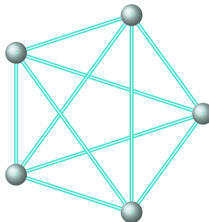
FIGURE 14.18 – Graphe K_5 : saurez-vous trouver des cycles hamiltonien et eulérien de ce graphe?
