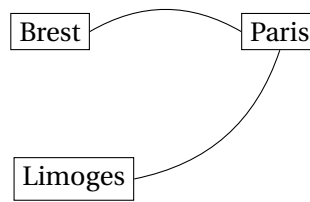
FIGURE 14.10 – Graphe d'ordre trois, de taille deux et de séquence [1, 1, 2]
