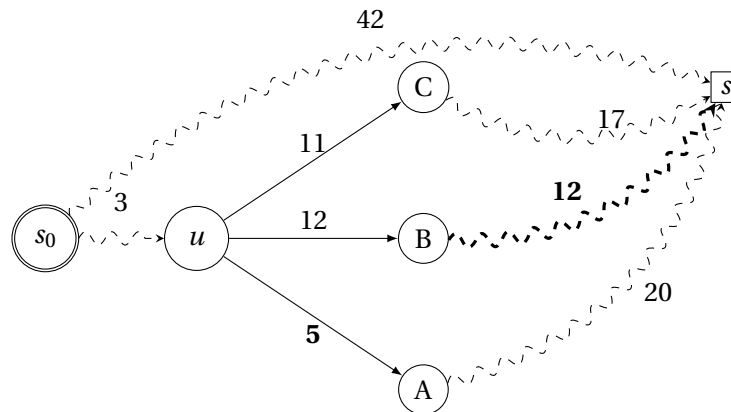
FIGURE 22.3 – Illustration du principe d’optimalité et de sous-structure optimale : trouver le plus court chemin dans un graphe orienté et pondéré. Les lignes droites sont des arcs. Les lignes ondulées indiquent les chemins connus dans le graphe : il faut imaginer qu’on n’a pas représenté tous les sommets. Les nombres représentent des distances ou les poids des arcs.
