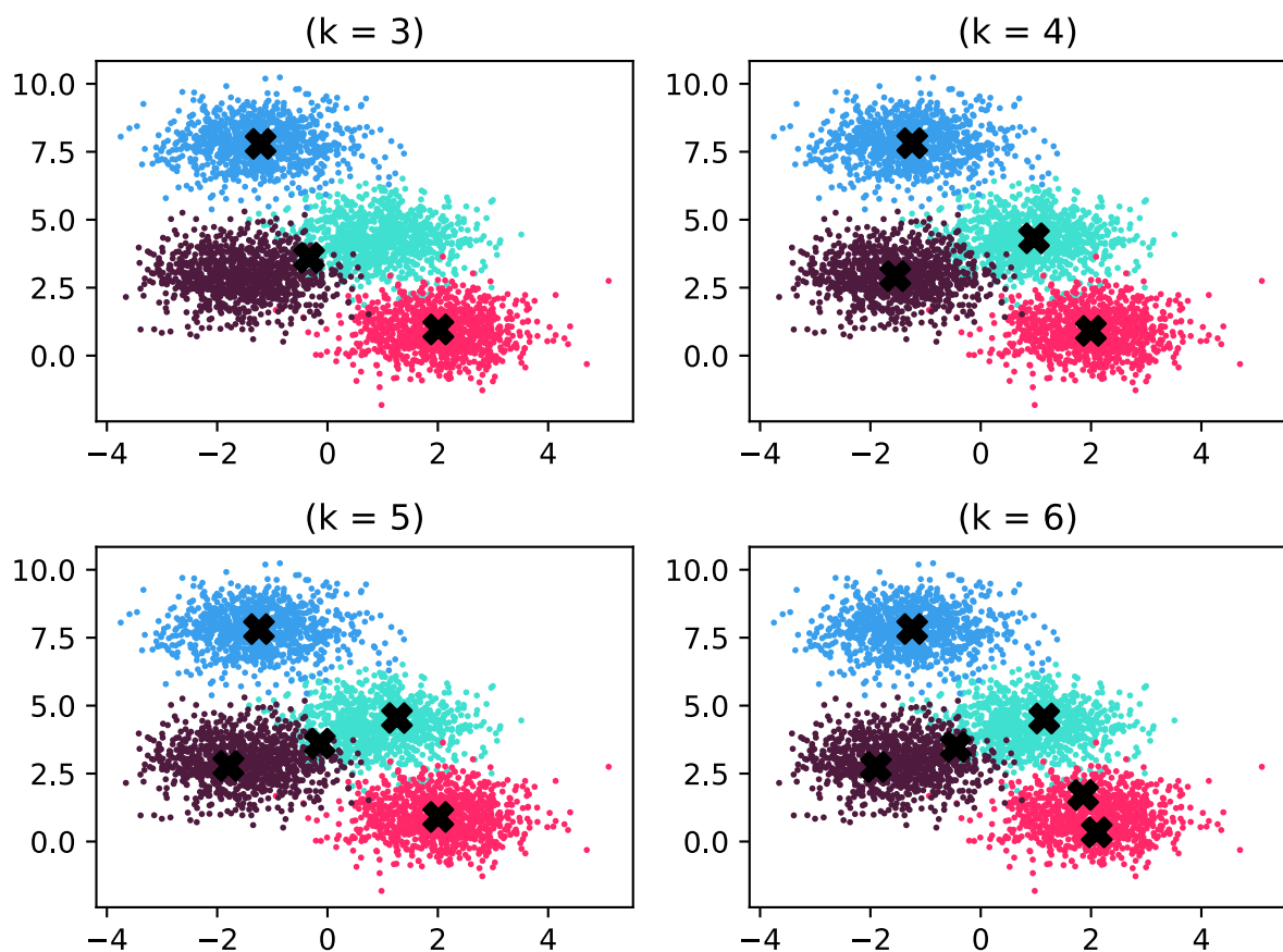
FIGURE 25.6 – Illustration des conséquences du choix du paramètre k dans k -moyennes. Sur cet exemple, seules quatre classes existent dans les données. k varie entre 3 et 6. Les barycentres sont représentés par des croix noires.
