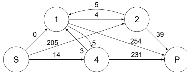
Figure 12 - Exemple de graphe résiduel
